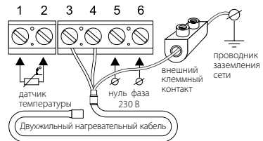
Схема подключения к 3-х проводной электрической сети
